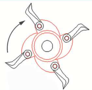
Speciale rotore ANTIURTO per ridurre i danni causati da urti Unique ANTI SHOCK rotor design to reduce damages when hitting hard objects
