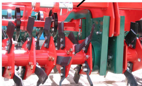
Helicoidal flanges for maximum cultivation across the full width Flange elicoidali per la massima lavorazione su tutta la larghezza
